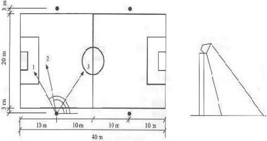
Mini futbol sahası aydınlatma detayları
