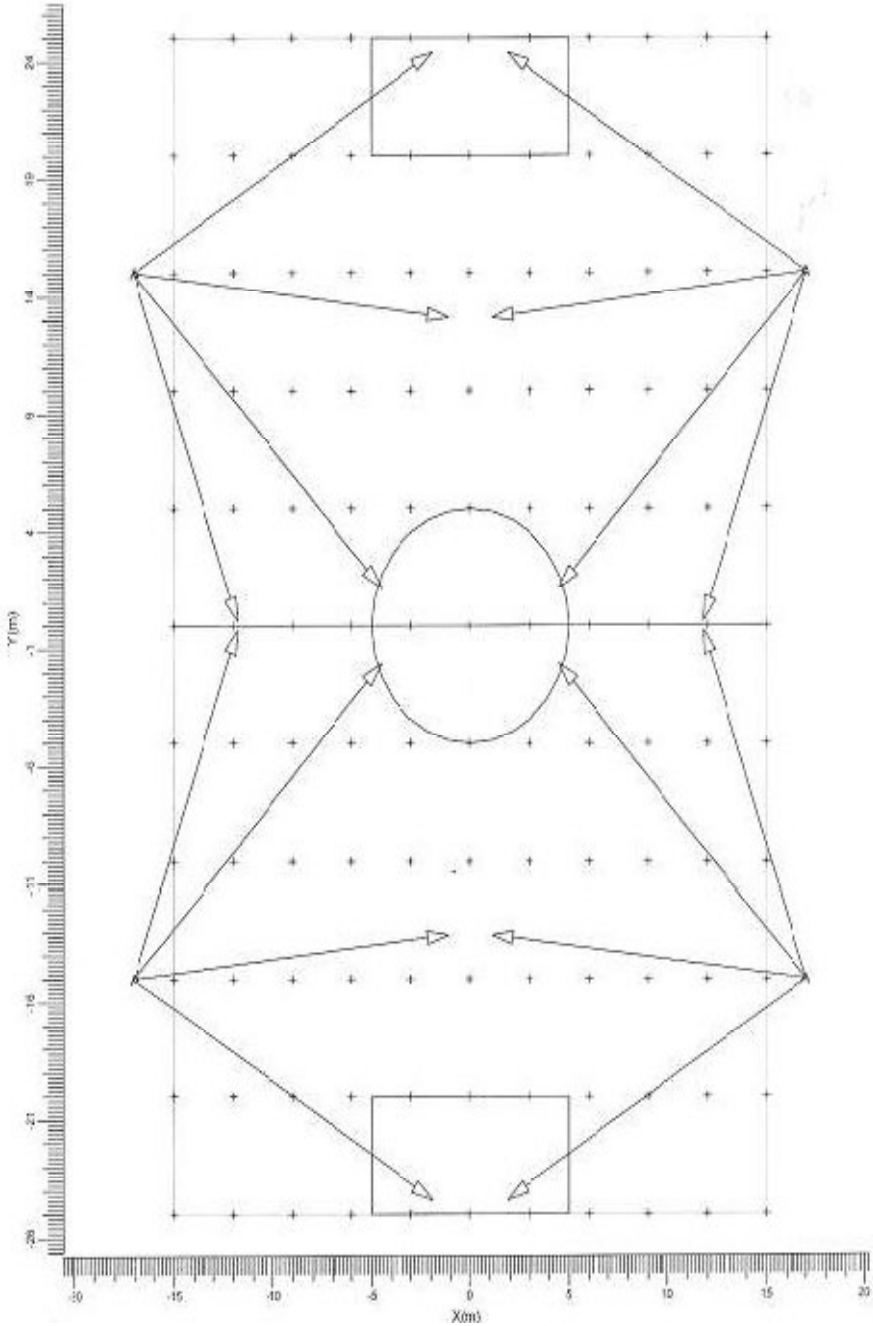
Bilgisayar programıyla yapılmış mini futbol sahası projesinin 16 adet projektörün aydınlatma noktalarını üstten gösteren kısmı
