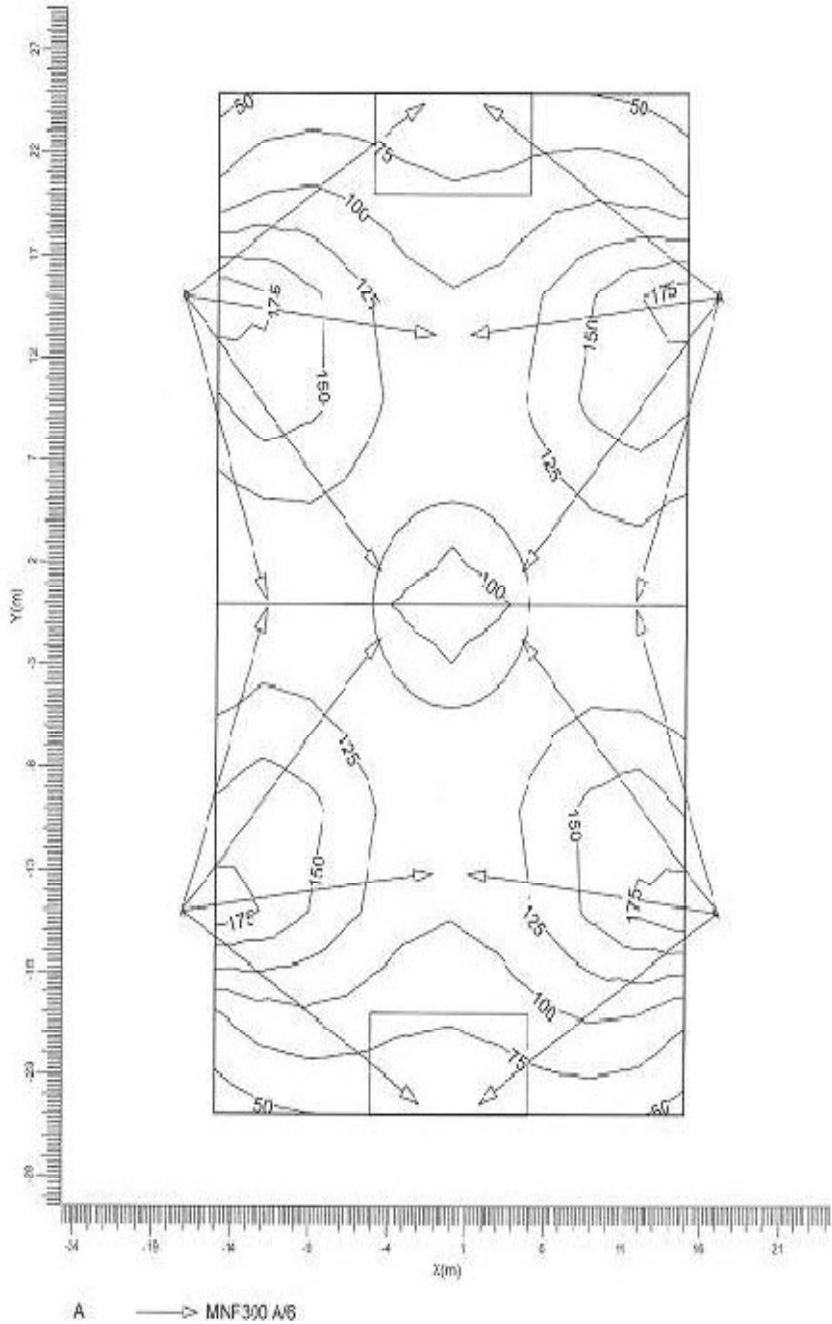
Bilgisayar programıyla yapılmış mini futbol sahası projesinin 16 adet projektörün aydınlatma noktalarını üstten gösteren kısmı
