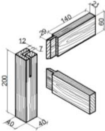
Őekil 2.8: Aık zıvanalı ayak kayıt birleřtirme Resim 2.10: Aık zıvanalı ayak kayıt birleřtirme
