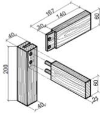
Şekil Hata! Belgede belirtilen stilde metne rastlanmadı..10: Kavelalı ve zıvanalı ayak kayıt birleştirme
